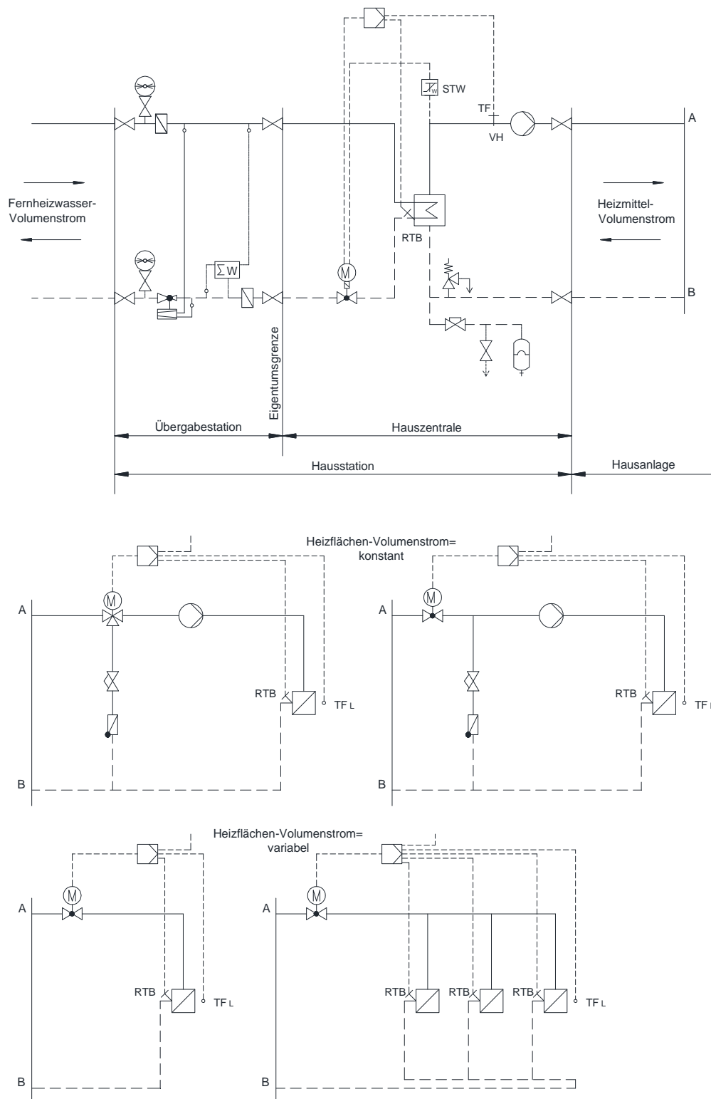
Bild 6: Hauszentrale-Raumluftheizung (RLH)
