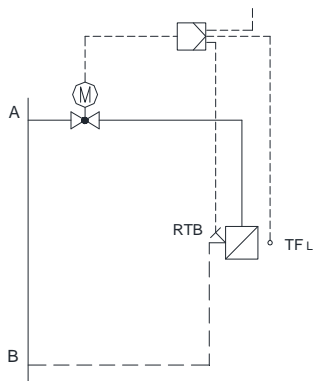
Bild 6a: Hauszentrale-Raumluftheizung (RLH)
