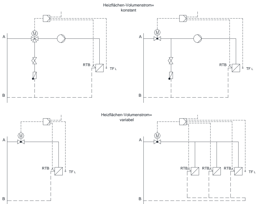
Bild 6b: Hauszentrale-Raumluftheizung (RLH)
