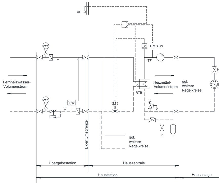
Bild 3: Hauszentrale-Raumheizung Prinzipschaltbild für den indirekten Anschluss
