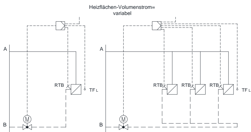
Bild 5: Hauszentrale-Raumluftheizung (RLH)
